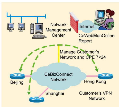
CeWebMon的拓扑结构
